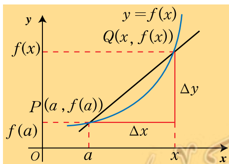
شكل (2) ميل الخط المقاطع \overrightarrow{PQ} هو: \frac{\Delta y}{\Delta x} = \frac{f(x) - f(a)}{x - a}
