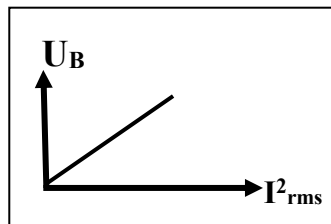
الطاقة المغناطيسية ومربع الشدة الفعالة للتيار
