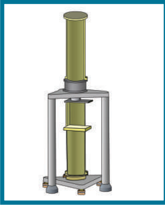
شكل 86 جرافيمتر
